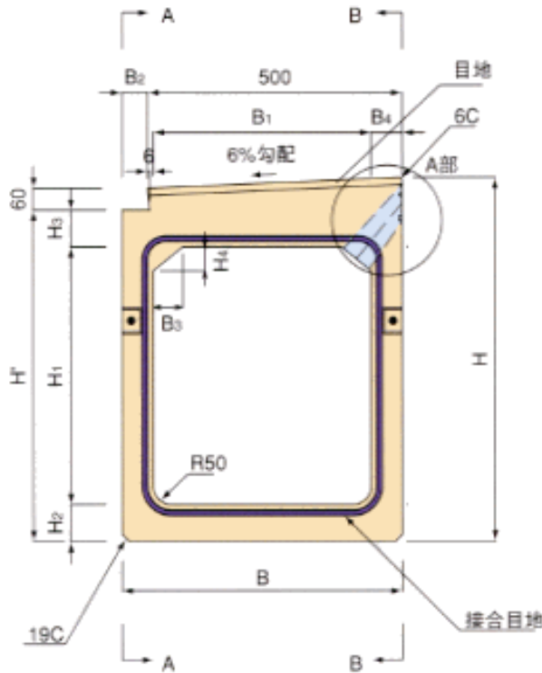
本体正面図
